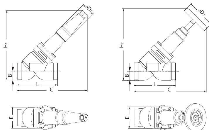
Прямые обратно-запорные клапаны SCA XXX STR
